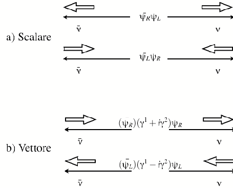
Figura 8.1: Stati con momento totale \mathbf{P} = 0 creati dal vuoto dalla densità scalare, (a), e vettoriale, (b). Le frecce sottili rappresentano la direzione della quantità di moto, le grandi la direzione dello spin. Gli elementi di matrice non nulli corrispondono alle regole enunciate nel testo per quanto riguarda gli operatori con chiralità definita, \psi_R e \psi_L .
