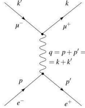
Figura 11.3: Rappresentazione grafica dell' ampiezza di annichilazione elettrone-positrone in coppie \mu^+ \mu^- . Le frecce indicano il flusso della carica elettrica negativa, quindi sono in direzione opposta ai momenti per e^+ e \mu^+ , q^\mu é il momento associato alla linea che rappresenta la propagazione del fotone. La quantità di moto si conserva nei vertici.
