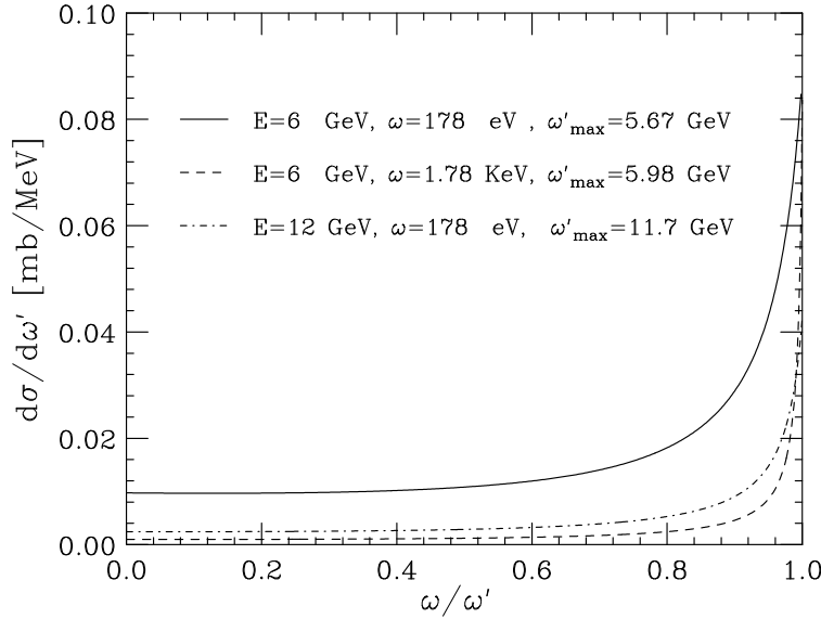
Figura 11.3: Distribuzione in energia di fotoni prodotti con diffusione Compton di elettroni relativistici.
