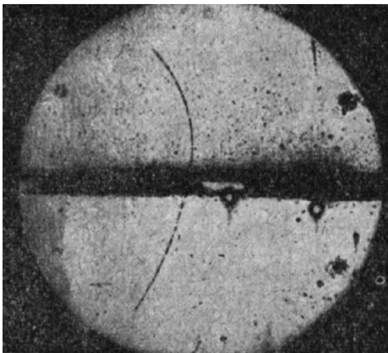
Figura 6.1: Foto di una camera a nebbia con una delle prime immagini di un positrone, C. D. Anderson, 1932. Il positrone si muove dal basso verso l'alto , come indicato dal fatto che la curvatura é inferiore nella parte alta della traiettoria, dovuto alla perdita di energia del positrone nell' attraversare la lastra di piombo, visibile in sezione a metà della camera. Da questa informazione si deduce che la carica della particella é positiva , mentra la massa é consistente con la massa di un elettrone.
