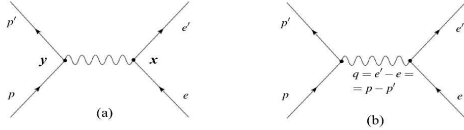
Figura 11.2: Rappresentazione grafica dell' ampiezza di diffusione elettrone-protone nello spazio tempo, (a), e nello spazio dei momenti, (b).
