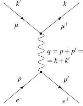
Figura 11.4: Rappresentazione grafica dell' ampiezza di annichilazione elettrone-positrone in coppie \mu^+ \mu^- . Le frecce indicano il flusso della carica elettrica negativa, quindi sono in direzione opposta ai momenti per e^+ e \mu^+ , q^\mu è il momento associato alla linea che rappresenta la propagazione del fotone. La quantità di moto si conserva nei vertici.
